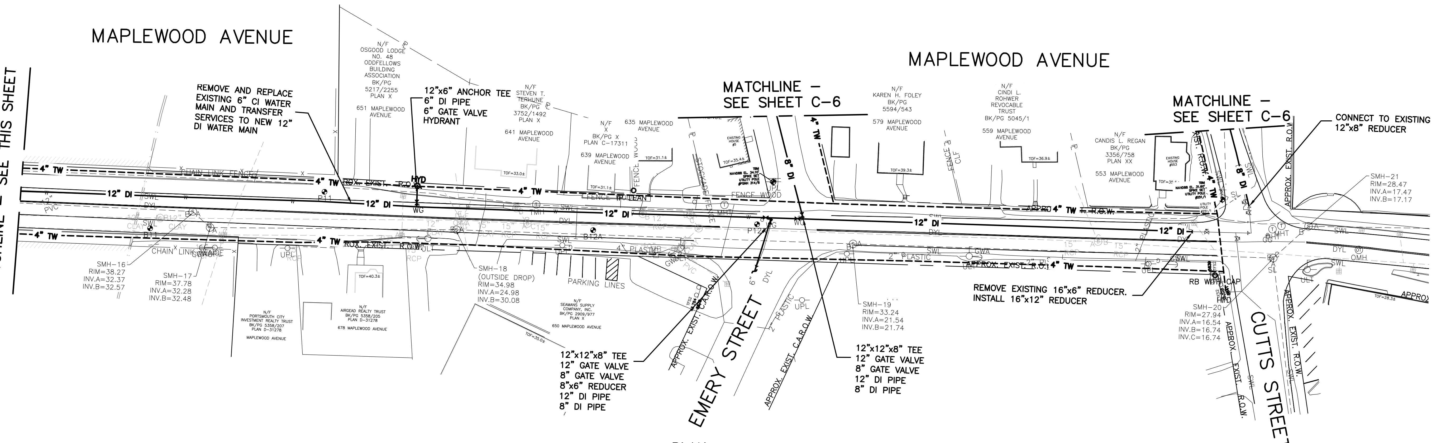
PLAN SCALE: 1" = 40'
